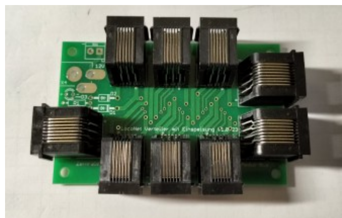
Loconet T Loconet-RJ45-Verteiler mit RJ12-Abgängen Durchschleifen mit RJ45 - Verteilen auf Handregler mit RJ12
